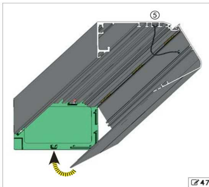
Instalación del cárter.
