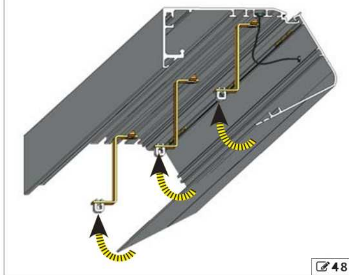
Instalación con costados laterales y estribo central.
