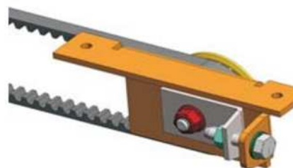
Polea de inversión
